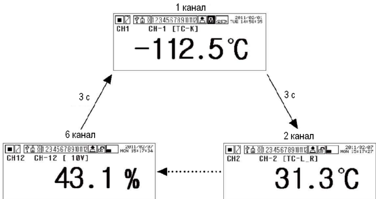
Индикация одного канала 1-6 каналы
