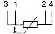
Схема 4 - четырёхпроводная
