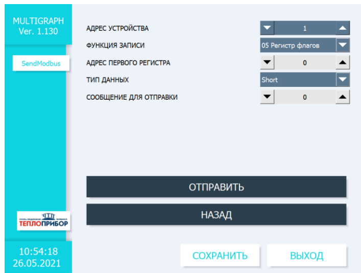
Рисунок 2.59 – Отправка Modbus-команды
